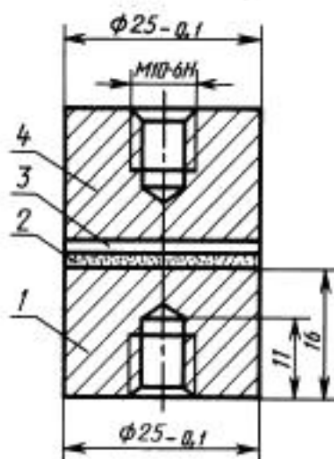
1 — образец; 2 — покрытие; 3 — клеящая прослойка; 4 — контробразец
