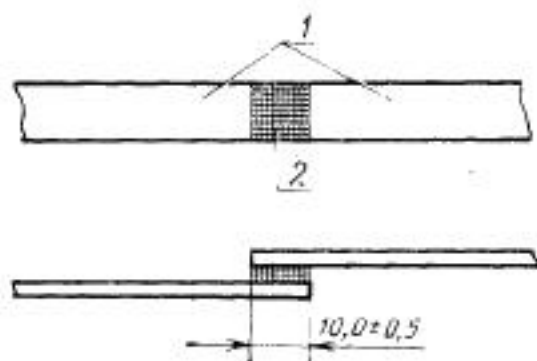
1—склеиваемый материал; 2—клеевое соединение
