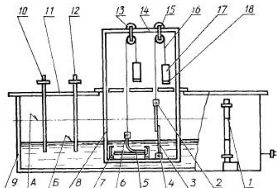
1—уровнемер; 2, 5—верхний зажим для образца; 3, 5—образец; 4, 7—нижний зажим для образца; 8—каркас; 9—камера для испытаний; 10—электроконтактный термометр; 11—крышка; 12—стеклянный термометр; 13—каретка; 14—направляющая каркаса; 15—ролик; 16—металлический трос; 17—груз; 18—платформа для груза; А—уровень жидкости по методу А; Б—уровень жидкости по методу Б
